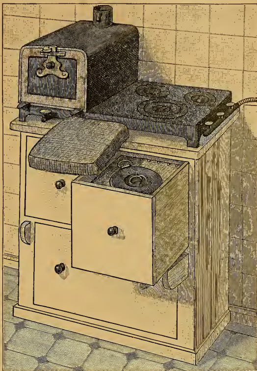
Fig. 11. Kochkistenschrank.
